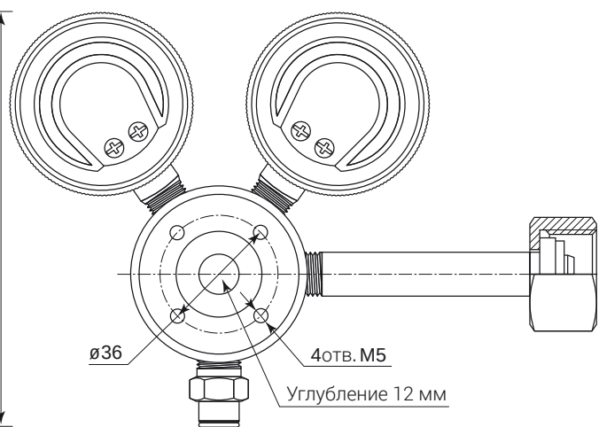
RPA1C, RPB1C - вид сзади
