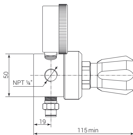
RPA1C, RPB1C - вид сзади
