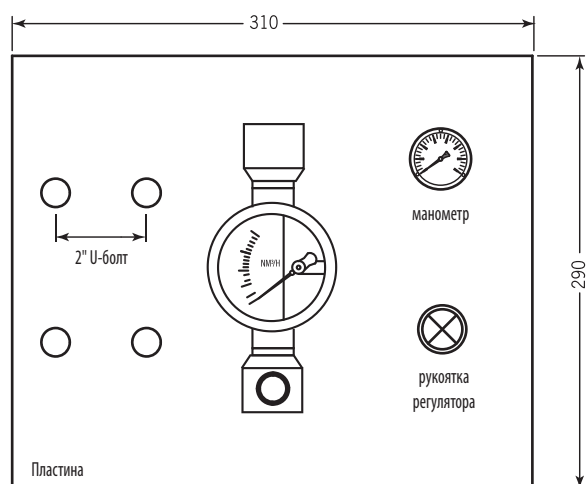
Тип G. Металлический расходомер - Одна линия
