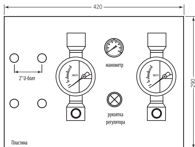
Тип G. Металлический расходомер - Две линии
