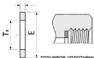
торцевое уплотнение для штуцеров типа AFC-G
